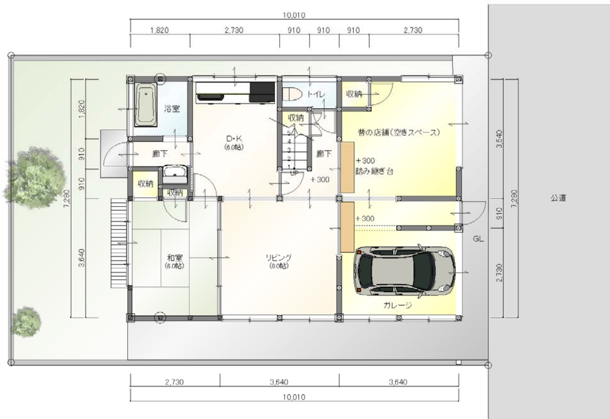
1F平面図
