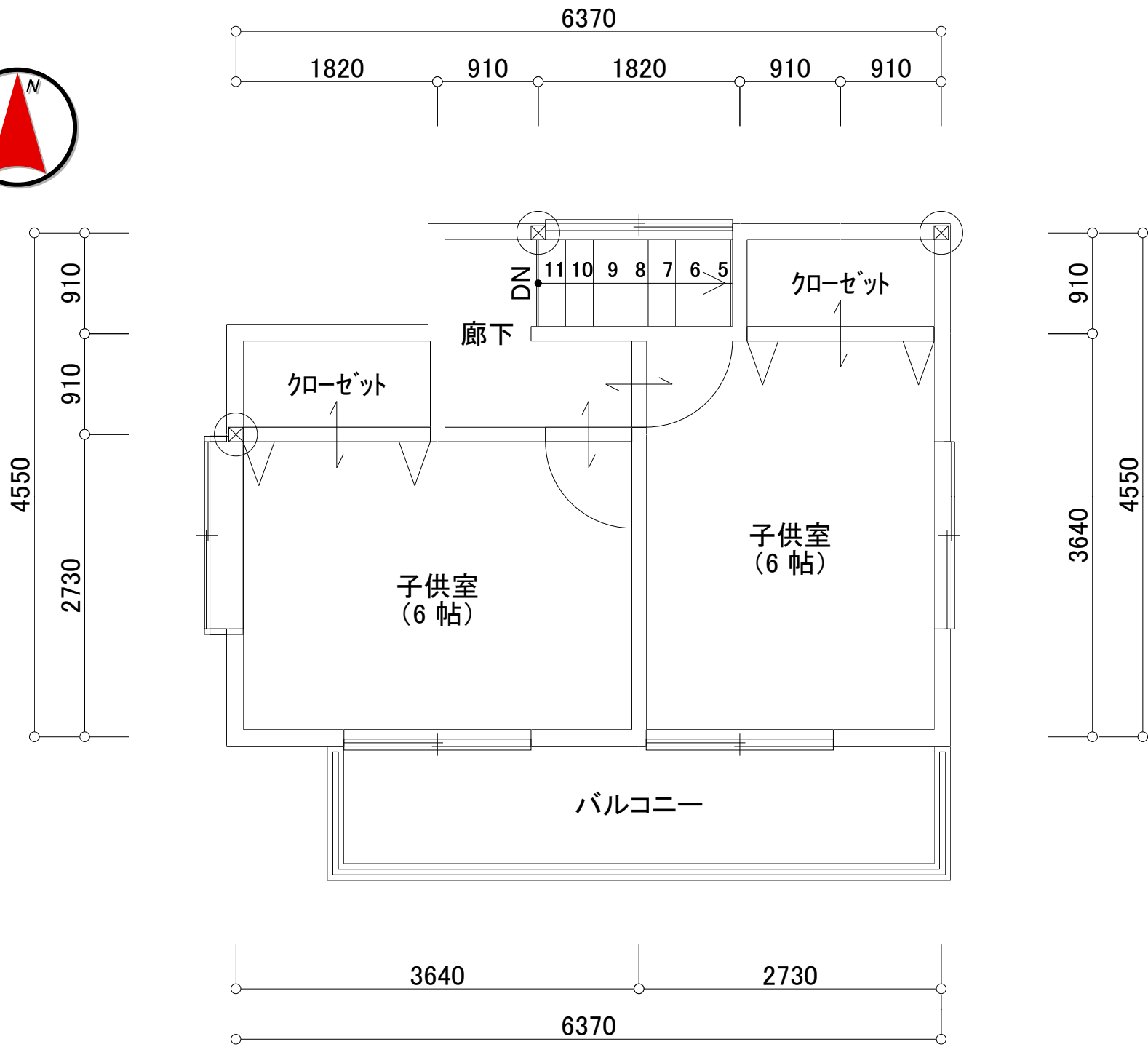
課題 2F平面図
