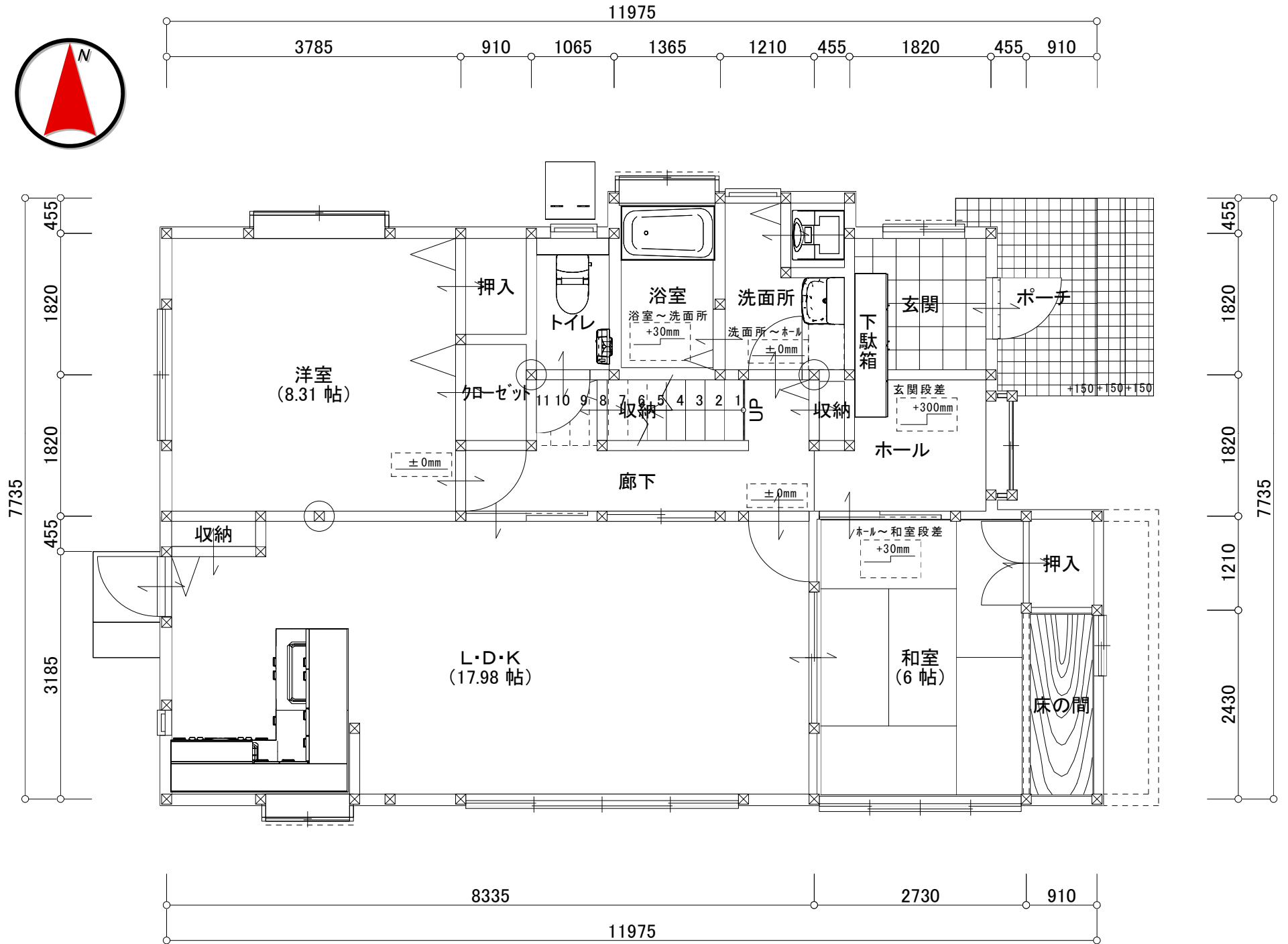
課題 1F平面図
